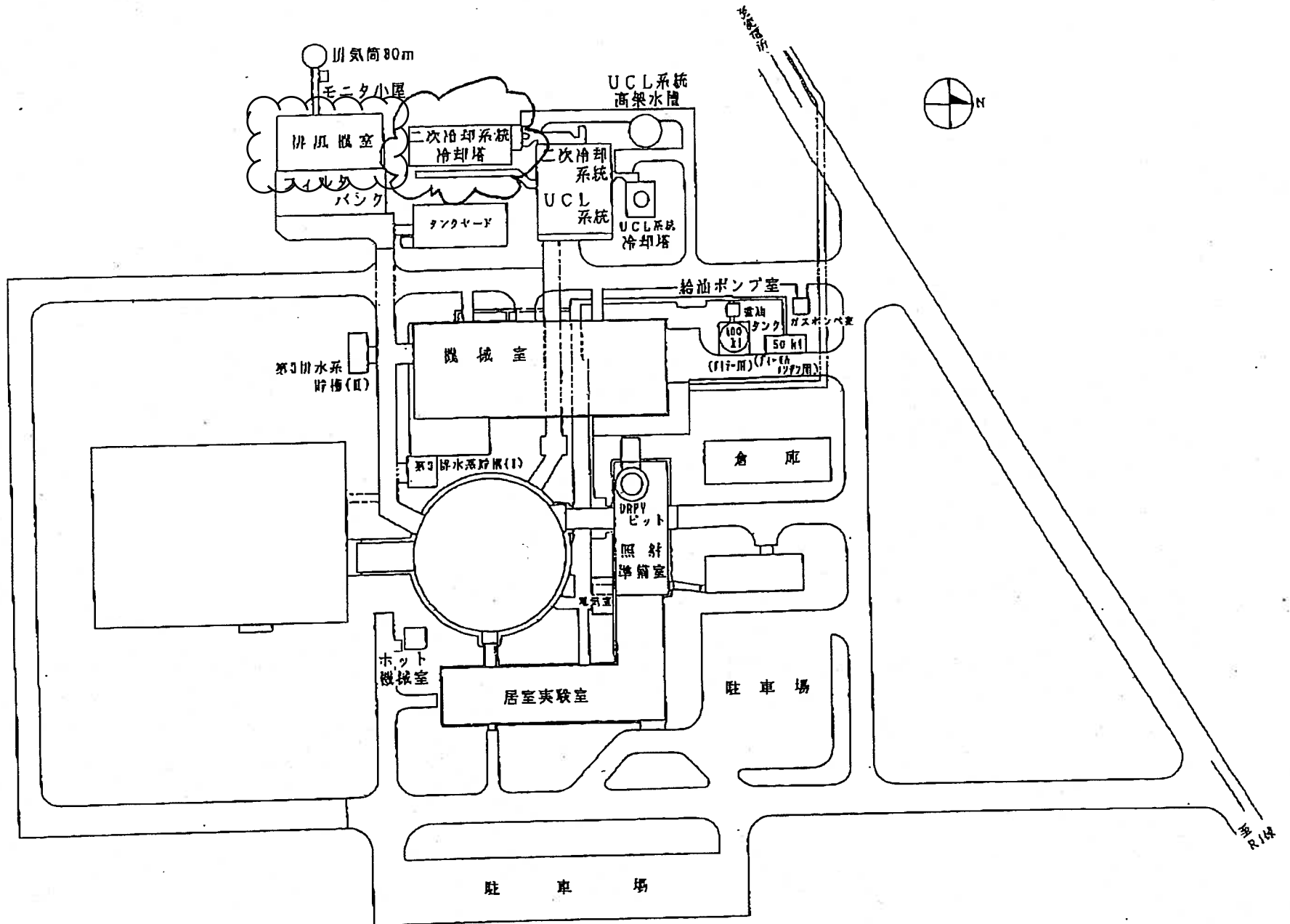
第1図 JMTR建家配置図
